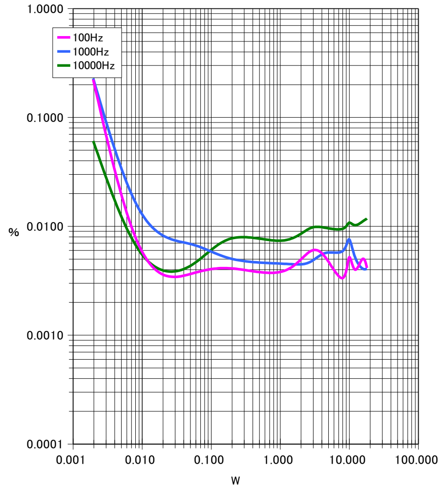
歪率特性カーブ
