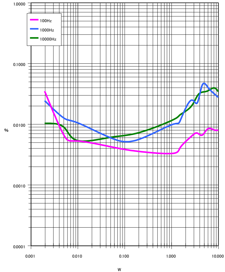
歪率特性カーブ
